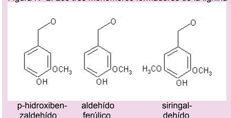
Figura N° 2. Los tres monómeros formadores de la lignina
